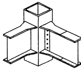
(a) 梁端扩大形连接
