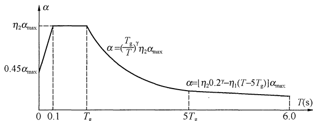
图 5.1.5 地震影响系数曲线
