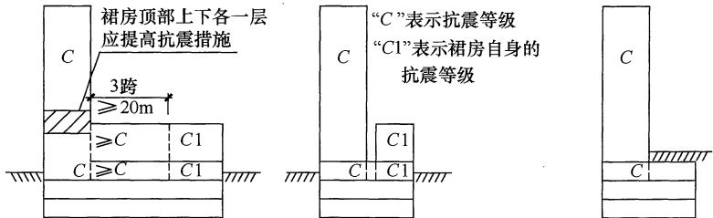
图 11 裙房和地下室的抗震等级
