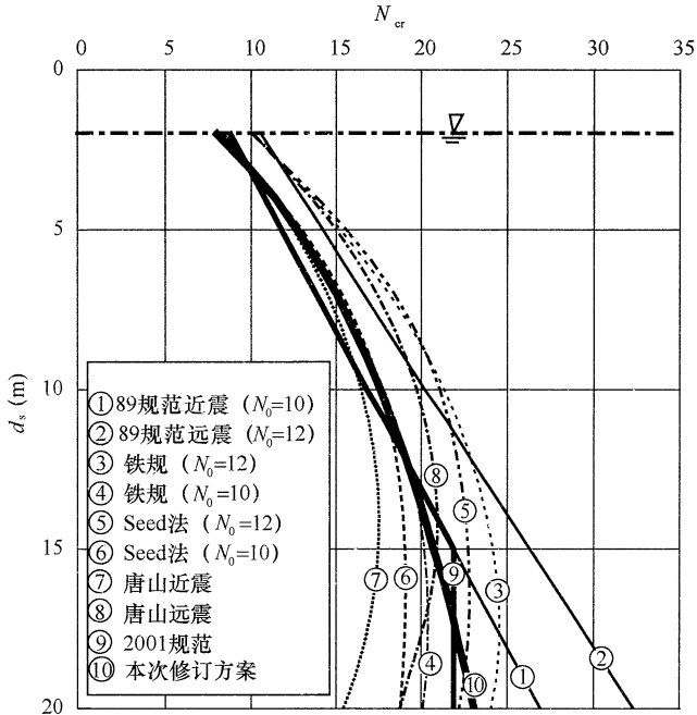
图8 不同方法液化临界值随深度变化比较 (以8度区为例)
